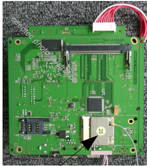
Half Length mini PCIe WiMax Module
